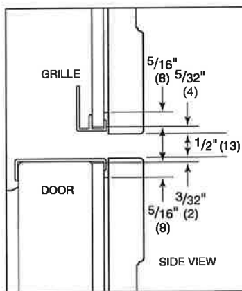
Grille Bottom / Door Top
